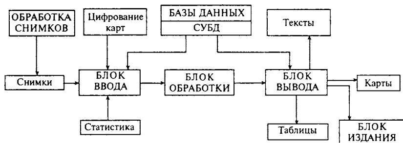
Рис. 14.4. Структура ГИС.
