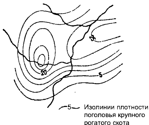
Рис. 4.7. Псевдоизолинии.
