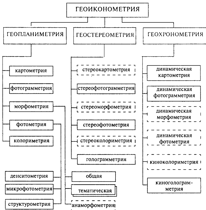
Рис. 17.3. Система геоикониметрии.
