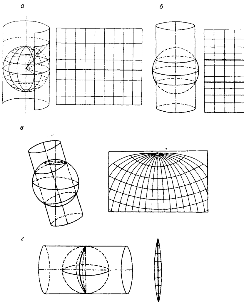
Рис. 3.6. Цилиндрические проекции.
