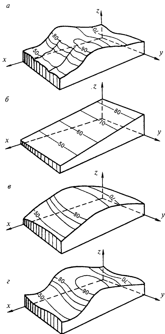
Рис. 12.16. Аппроксимации поверхностей:
