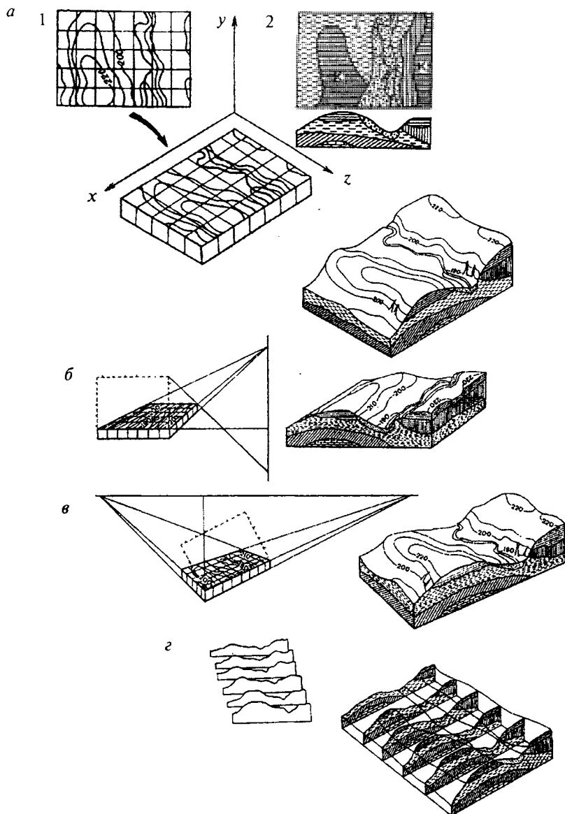
Рис. 12.8. Блок-диаграммы.
