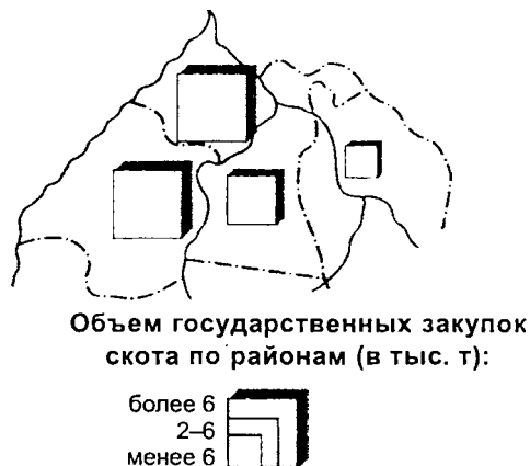
Рис. 4.15. Картодиаграмма.
