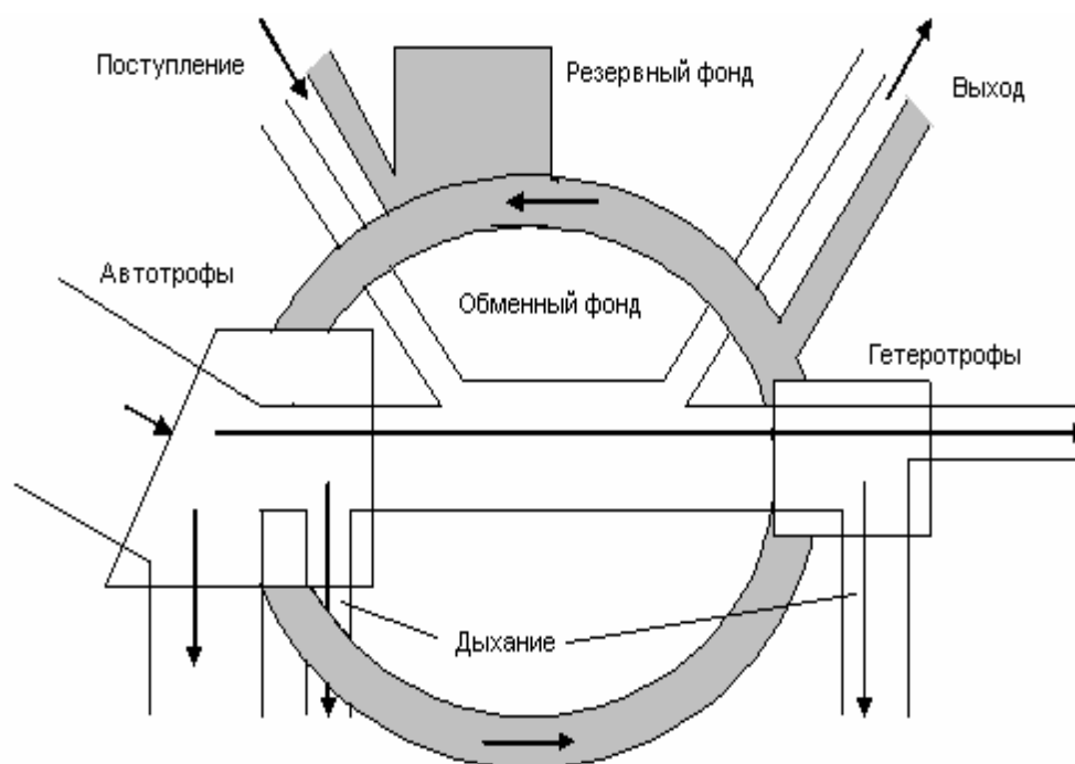
Рис. 10. Биогеохимический цикл на фоне упрощенной схемы потока энергии (по Одум, 1986. Т. 1. С. 202)
