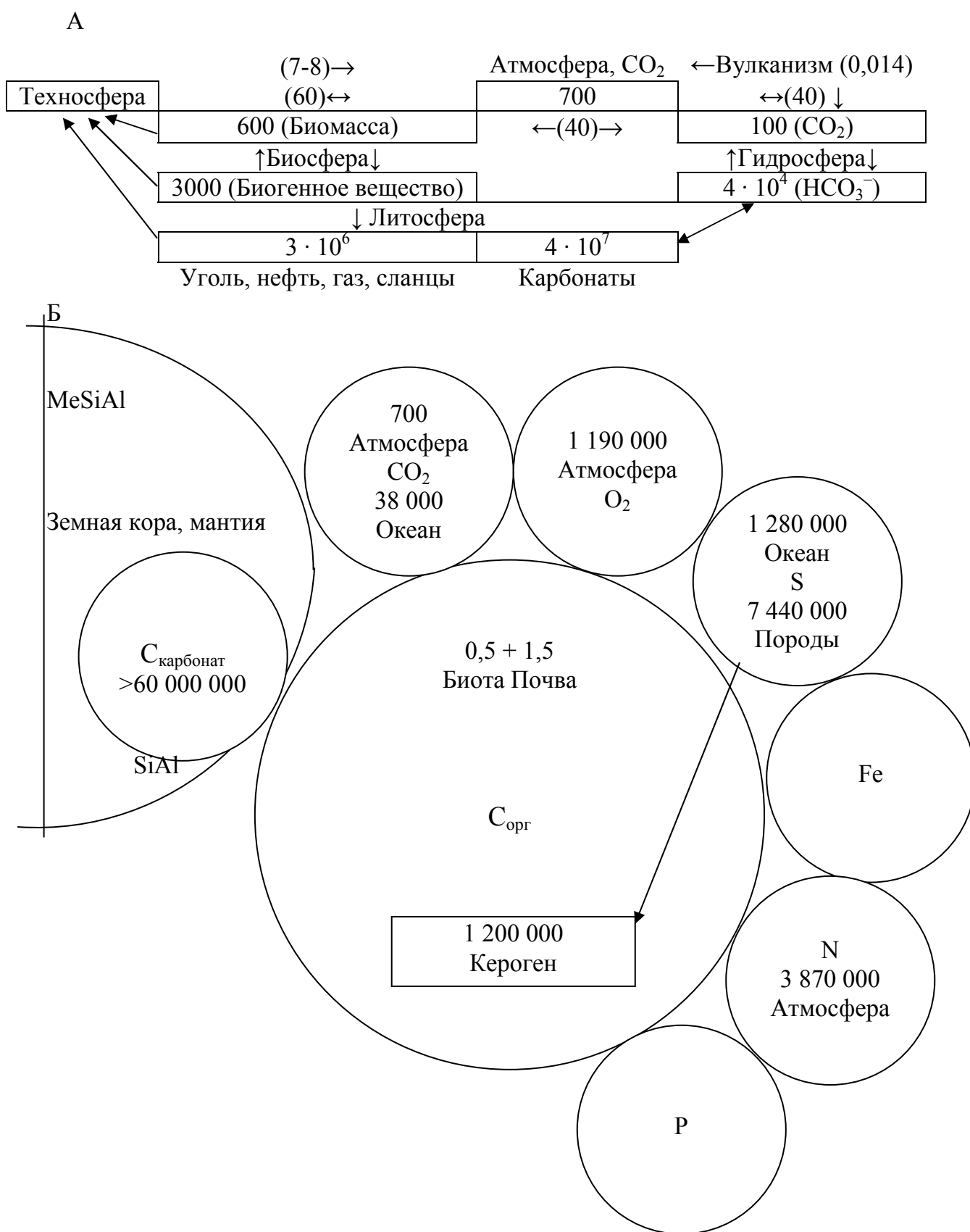
Рис. 12. Глобальный круговорот углерода:
