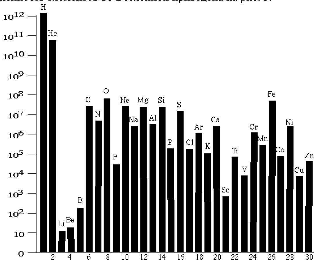
Рис. 5. Относительная распространенность элементов во Вселенной
