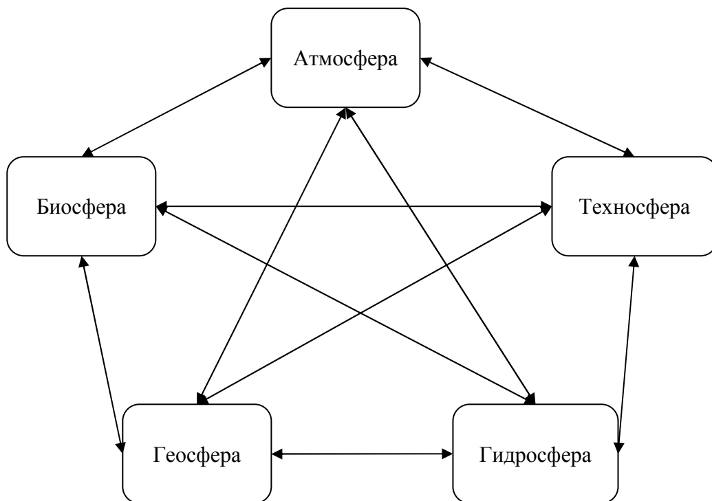
Рис. 16. Универсальная схема для описания циркуляции веществ между резервуарами Земли
