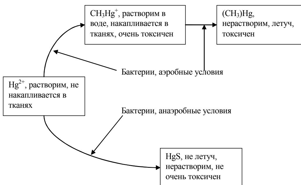
Рис. 20. Поведение ртути в водной среде (до аккумуляции организмами)
