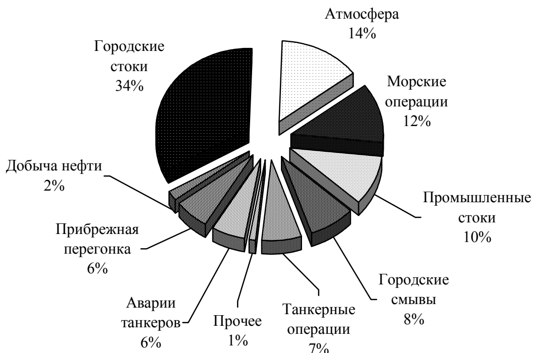
Рис. 18. Антропогенное поступление нефтепродуктов в океаны (Frid, 2002)
