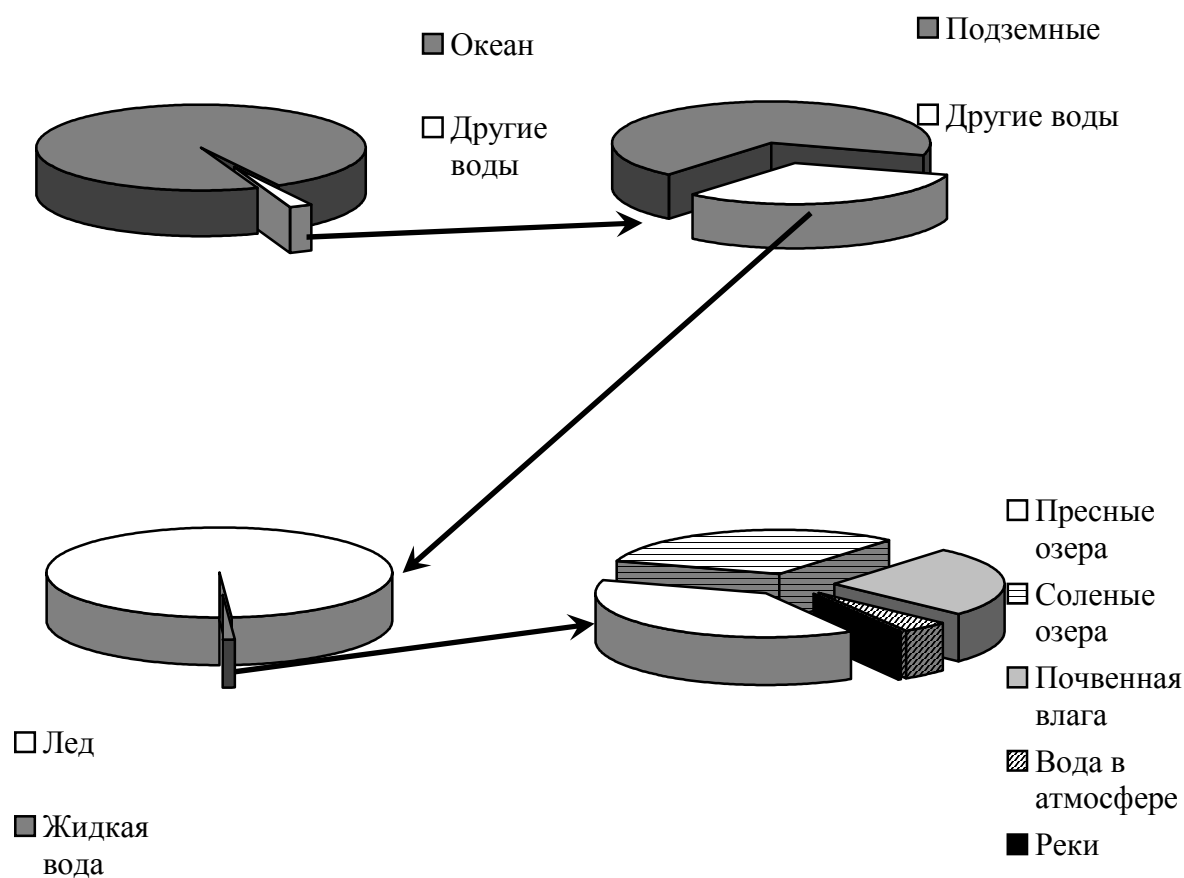
Рис. 8. Состав гидросферы по классам вод
