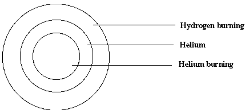
Рис. 1. Схематическое изображение Солнца
