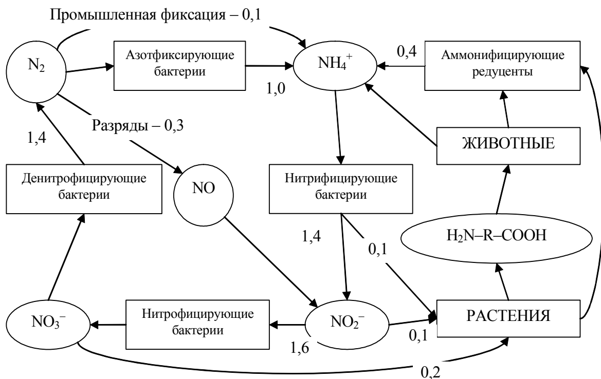
Рис. 13. Круговорот азота (в Гт·год -1 )
