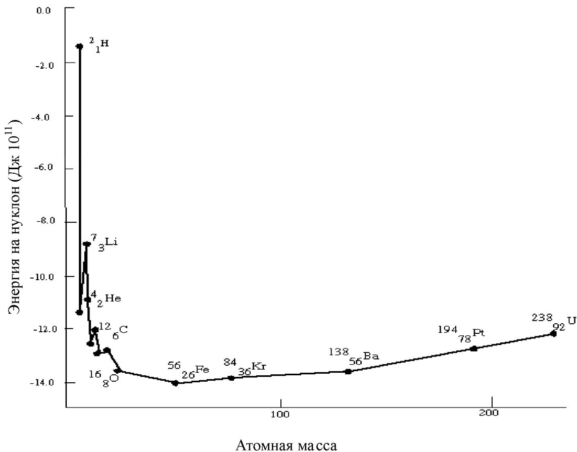
Рис. 4. Устойчивость ядер химических элементов
