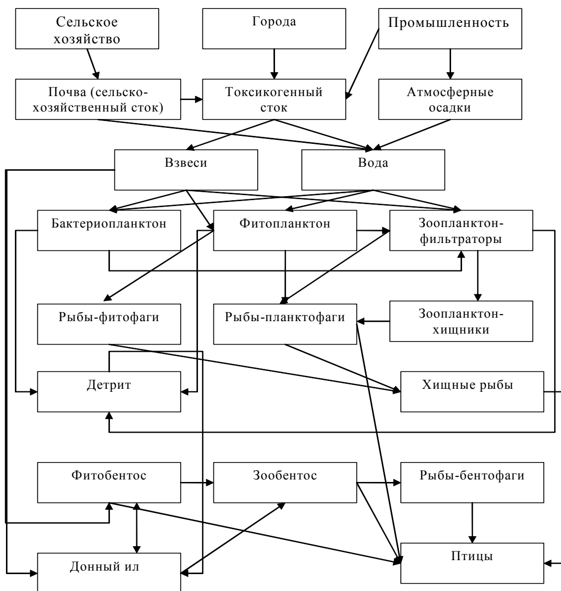
Рис. 19. Миграционные пути консервативных токсикантов в водных экосистемах
