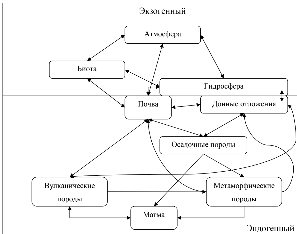
Рис. 9. Экзогенный и эндогенный циклы
