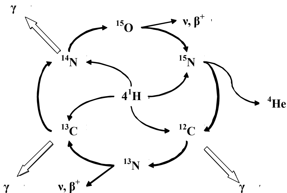
Рис. 2. Углеродный цикл Бете–фон Вайцекера
