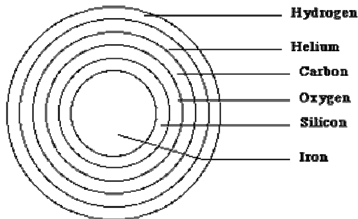
Рис. 3. Звезды вдвое (а), втрое (б) тяжелее Солнца и звезда перед взрывом сверхновой (в)
