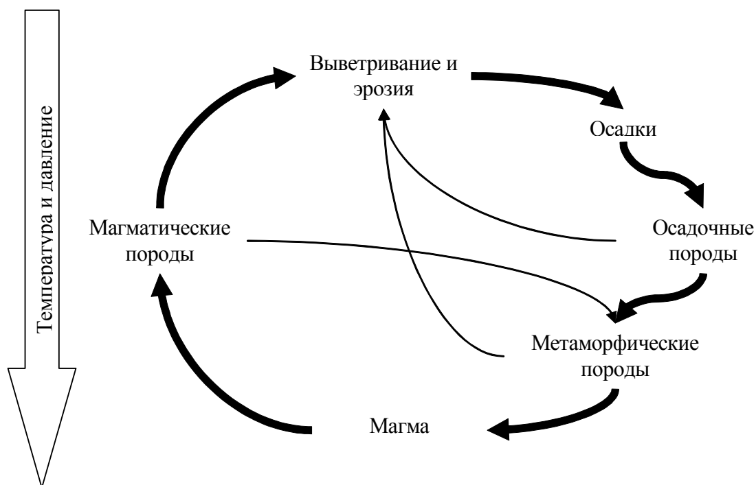
Рис. 7. Геологический цикл
