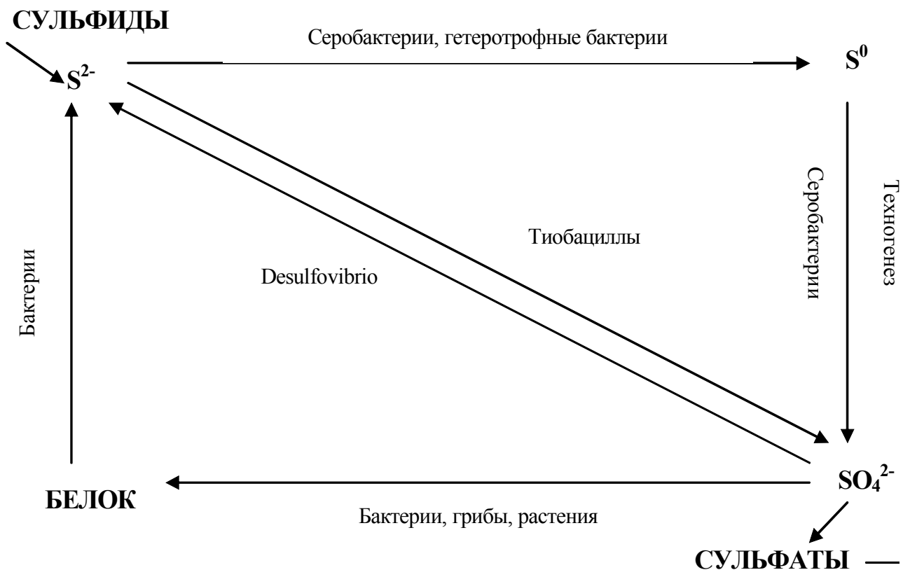
Рис. 15. Схема круговорота серы
