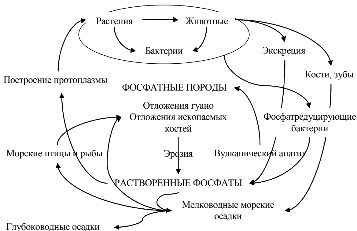
Рис. 14. Круговорот фосфора (по Одум, 1986. Т. 1. С. 210)
